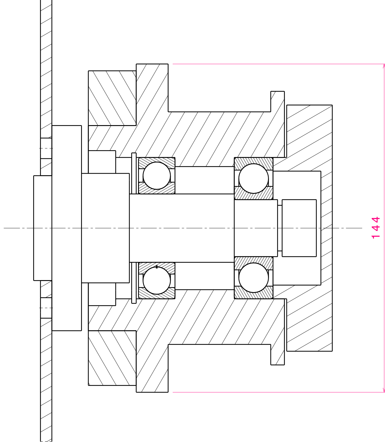
Coupe A-A Echelle : 1:1
